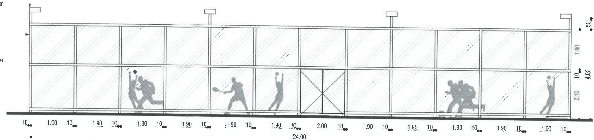
ELEVATIE TRONSON 1
