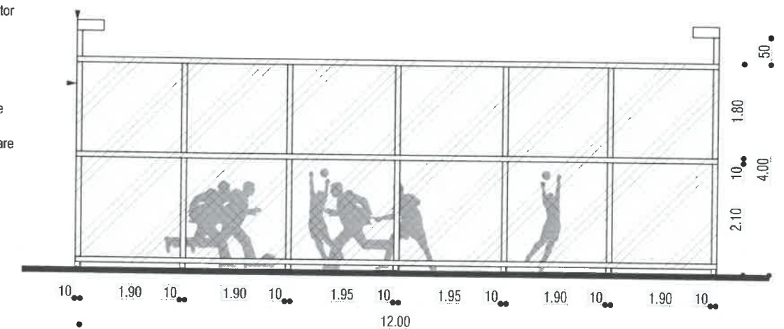
ELEVATIE TRONSON 2
