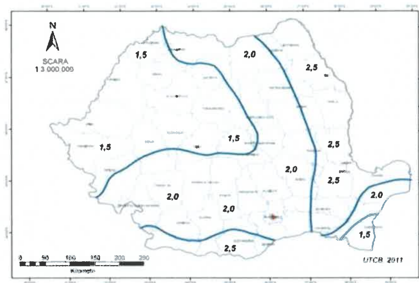
Figura 3.1 Zonarea valorilor caracteristice ale încărcării din zapada pe sol s_g , \text{kN/m}^2 , pentru altitudini A \leq 1000 m
