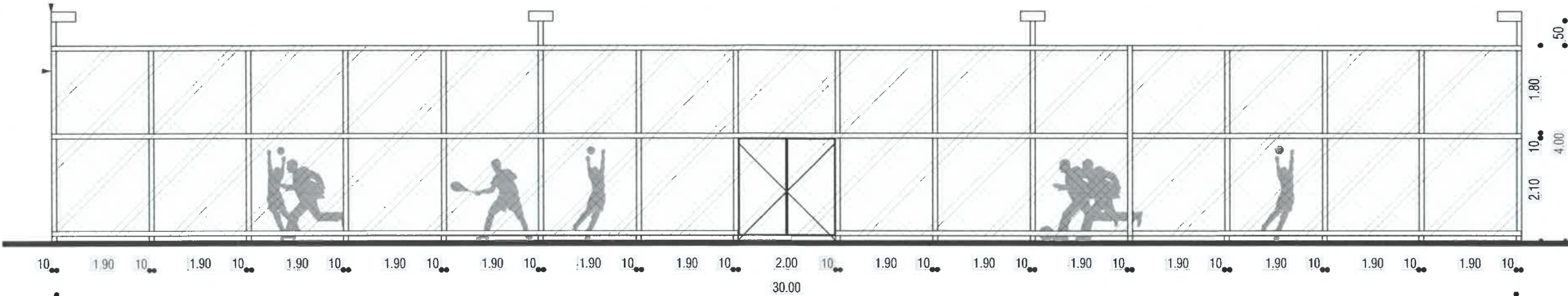
ELEVATIE TRONSON 1
