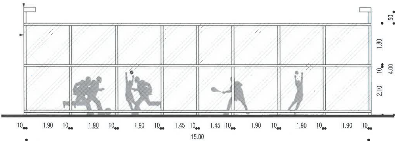
ELEVATIE TRONSON 2
