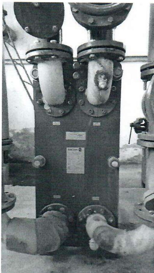
Foto 1 – Schimbatoare de caldura in placi din circuitul de incalzire
