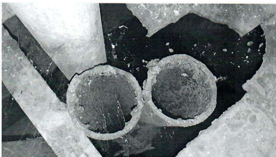
Foto 9 – Segmente de teava corodate extrase dupa avarii
