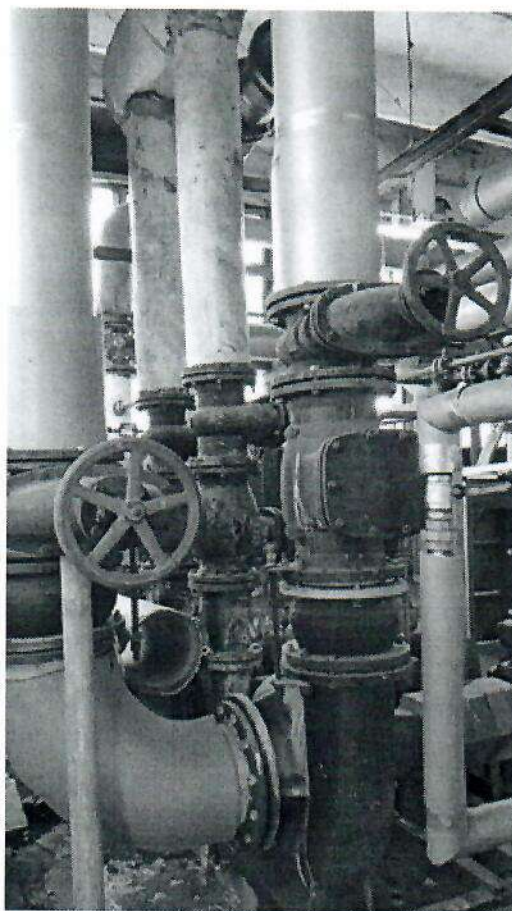
Foto 5 – Detalii cu armaturile din instalatie
