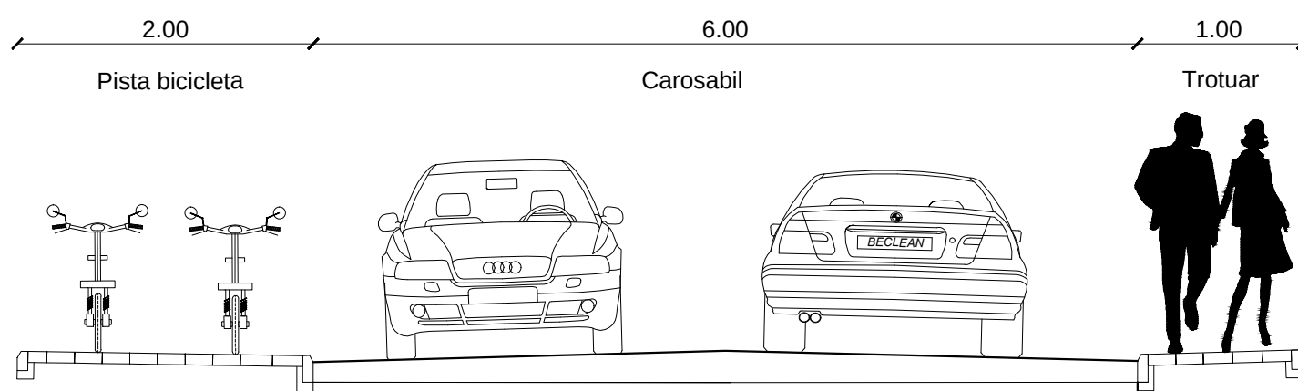
PROFIL TRANSVERSAL TIP 1 sc. 1:50
