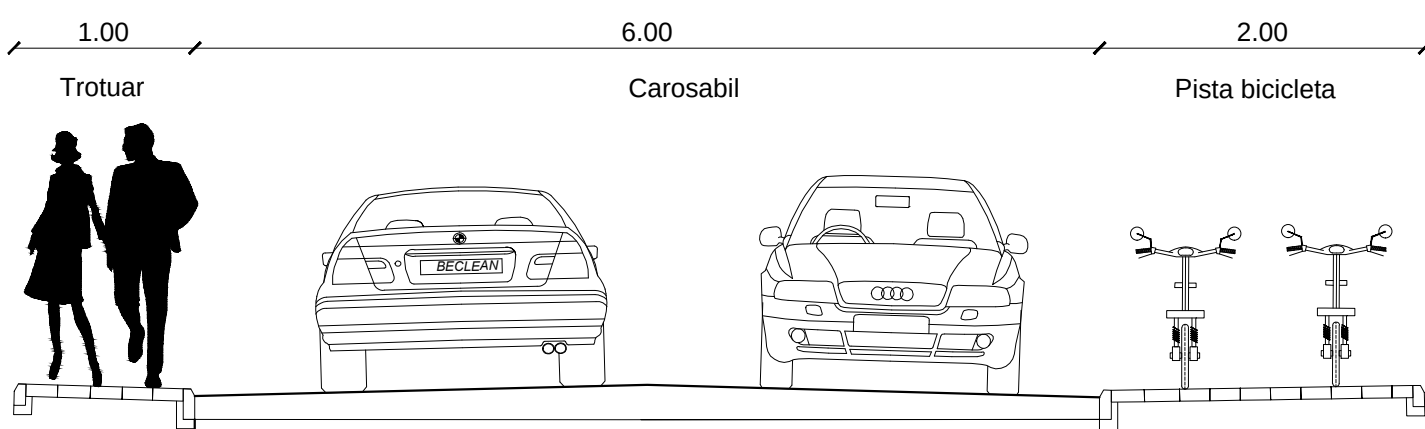
PROFIL TRANSVERSAL TIP 2
