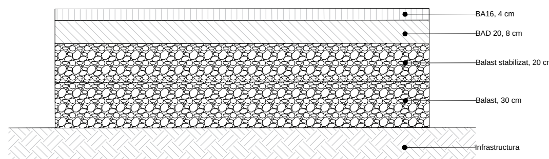
DETALIU DRUM PROPUS
