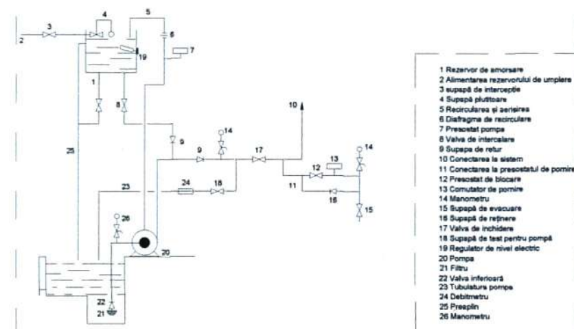
Fiecare pompă principală trebuie să fie echipată cu un rezervor de amorsare (capacitate = 500 litri)
