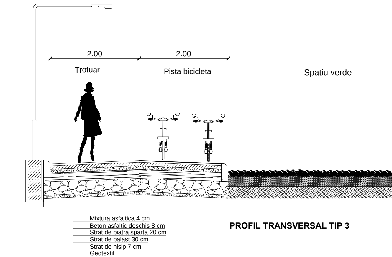
DETALIU TROTUAR CU PISTA BICICLETA sc. 1:50
