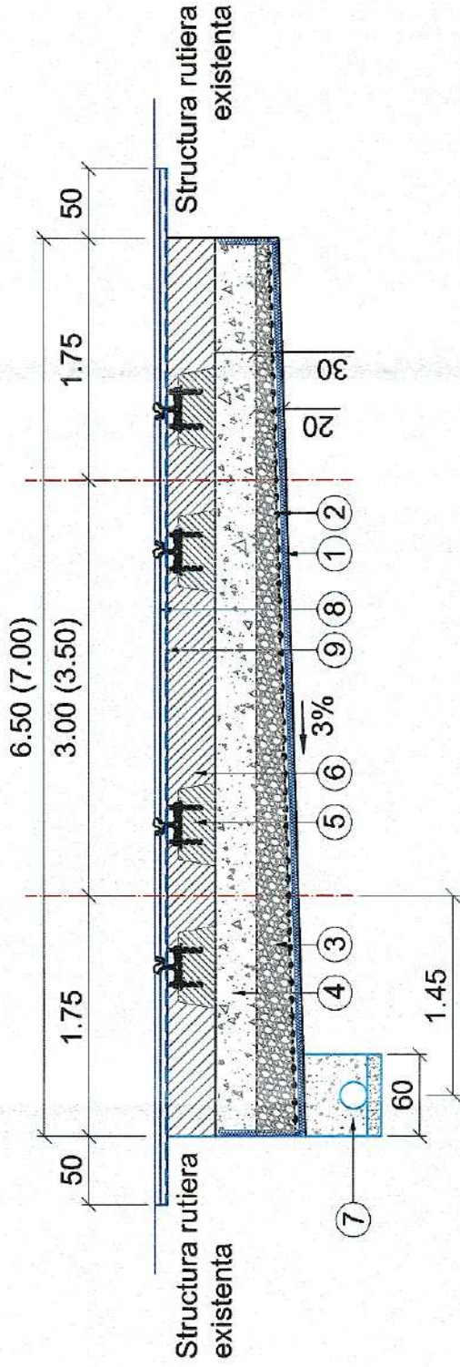
Linie dubla
