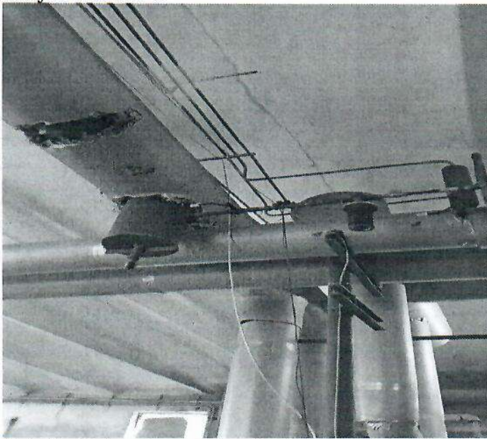
Foto 7 – Sistem de urmarire si reglare a presiunii din circuitul secundar
