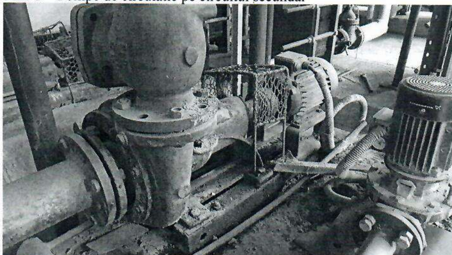
Foto 4 – Pompe de circulație pe circuitul secundar
