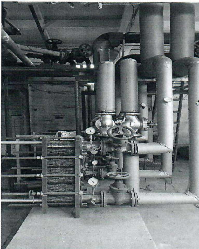
Foto 1 – Echipamentele termice din punctul termic
