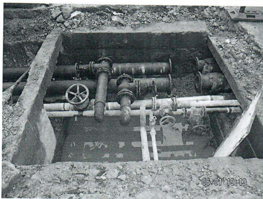
Foto 12,13 – Retele cu agenti termici secundari
