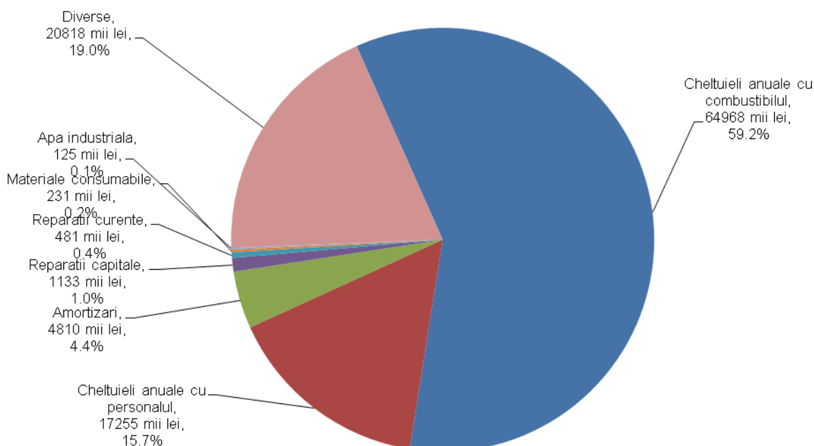
fig. 3.c - Structura cheltuielilor anuale ale CET Arad , în anul 2015, - valori în mii lei și % din cheltuielile anuale totale,- Cheltuieli anuale totale în anul 2015 = 109820 mii lei
