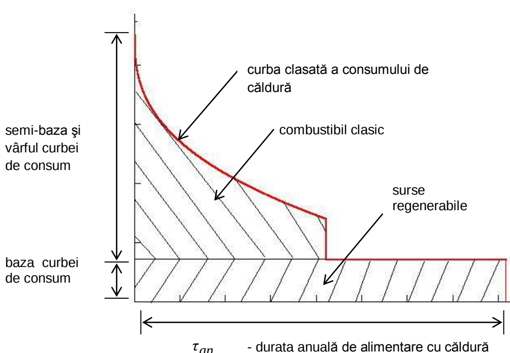
Fig. 2.i – Conceptul de utilizare a surselor regenerabile și combustibililor clasici, pentru asigurarea cererii urbane anuale de căldură a SACET urbane.
