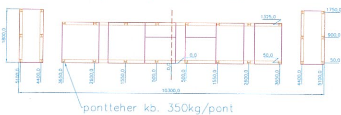
Metszet B (Alaprajz) (Statika / Súlyszámítás)
