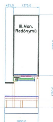
Metszet D (Oldal Metszet) VEDERE LATERALA
