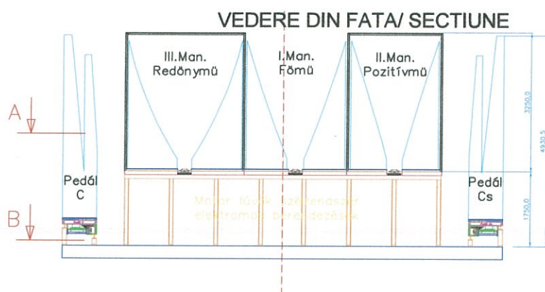
Metszet C (Szemből Metszet)
